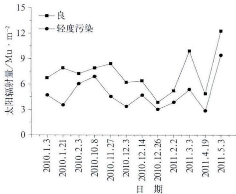
图 10 2010—2011 年空气质量对太阳辐射的影响
