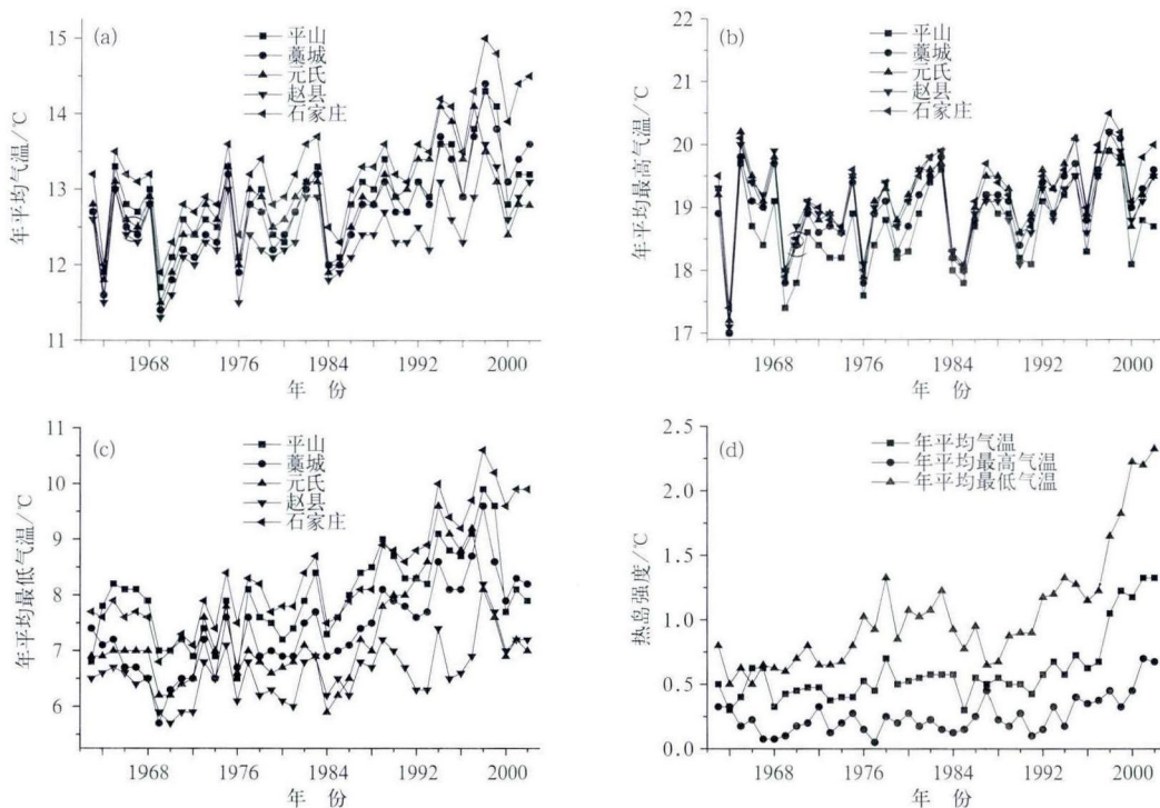
图 5 1963—2002 年石家庄、平山等 5 站的年平均气温(a)、年平均最高气温(b)、年平均最低气温(c)和同时段石家庄市热岛强度(d)变化图
