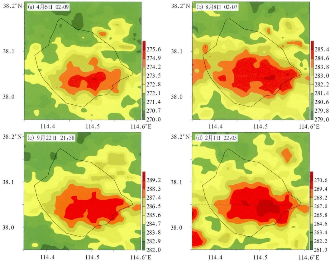
图 9 2011 年春、夏、秋、冬四季不同时段晚上地表温度分布图
