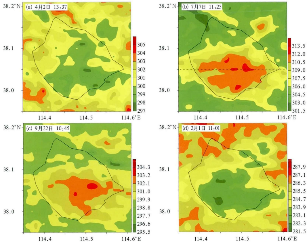
图 8 2011 年春、夏、秋、冬四季不同时次白天地表温度分布图
