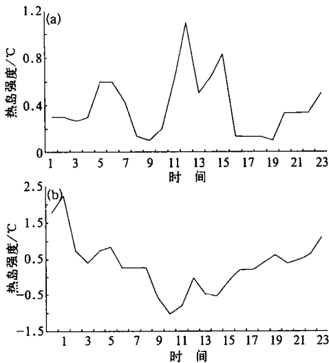
图 12 夏(a)、冬(b)两季热岛强度 随时间变化图
