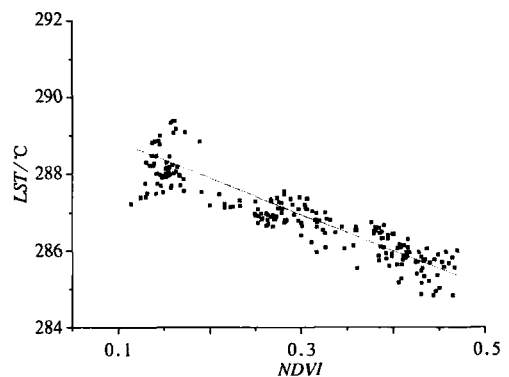
图 17 LST 与 NDVI 之间的关系
