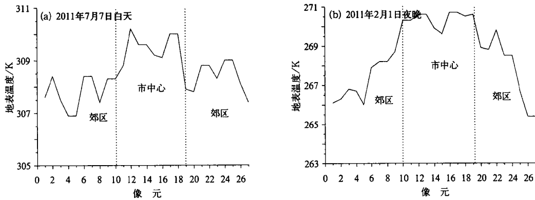
图 11 夏季白天(a)、冬季晚上(b)地表温度剖面分析图(X轴)
