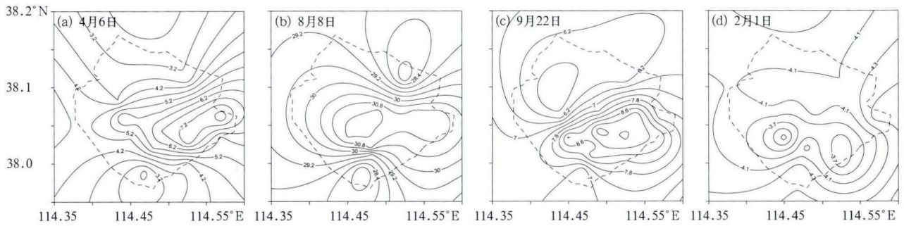
图 7 2011 年春、夏、秋、冬四季不同时次晚上气温空间分布图
