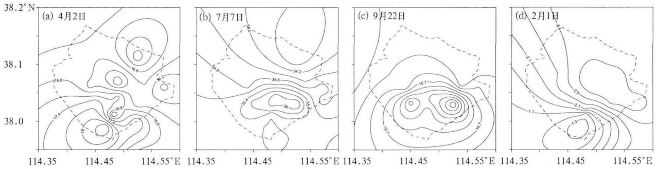
图 6 2011 年春、夏、秋、冬四季不同时次白天气温空间分布图
