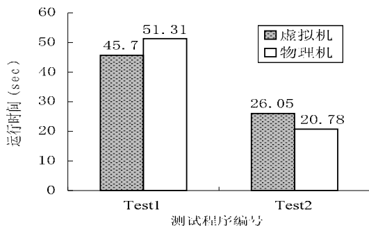
图 6 CPU 性能测试对比图
