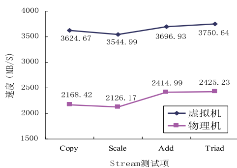
图 7 Memory 性能测试对比图
