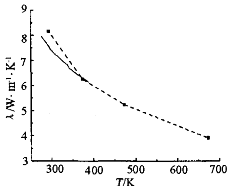
图 2 Nd:GGG 晶体导热系数
