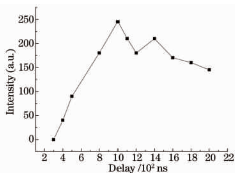
图 3 钾 769.90 nm 谱线的衰减特性
