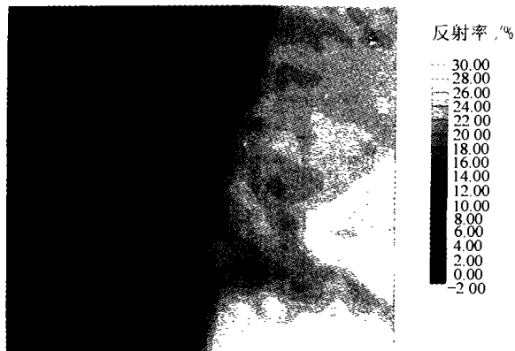
图 2 0.865 \mu\text{m} 波段 SeaWiFS 反射率等值线图 Fig.2 The isoline of reflectance at SeaWiFS 0.865 \mu\text{m} band
