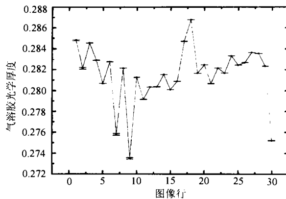
图 5 图像中每行气溶胶平均光学厚度与标准偏差 Fig.5 The average aerosol optical thickness and the standard deviation
