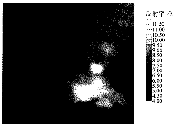
图 3 0.55 \mu\text{m} 波段 SeaWiFS 反射率等值线图 Fig.3 The isoline of reflectance at SeaWiFS 0.55 \mu\text{m} band
