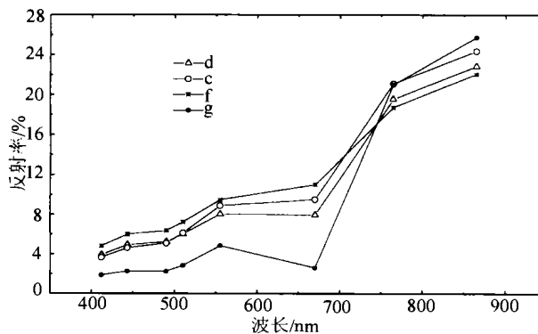
图 6 图 1 所标示陆地像元 SeaWiFS 8 波段反射率曲线 Fig.6 The reflectance curve of land surface as Fig.1 mark
