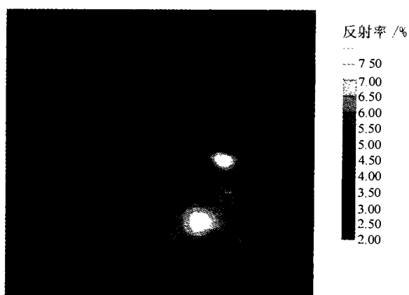
图 4 0.443 \mu\text{m} 波段 SeaWiFS 反射率等值线图 Fig.4 The isoline of reflectance at SeaWiFS 0.443 \mu\text{m} band
