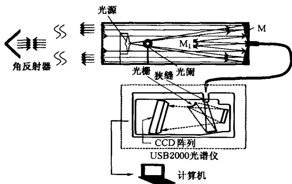
图 1 DOAS 系统结构图
