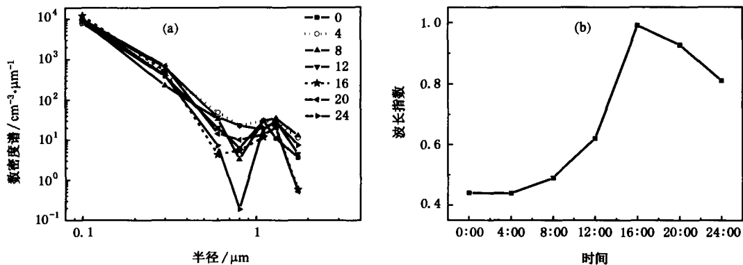
图 5 (a)2005 年 10 月 9 日一天中 0,4,8,12,16,20,24 点的粒谱分布,(b)为对应时间的波长指数的变化
