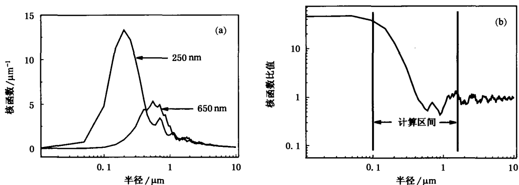
图 2 (a)250nm 和 650nm 上的核函数,(b)250nm 和 650nm 上的核函数比值
