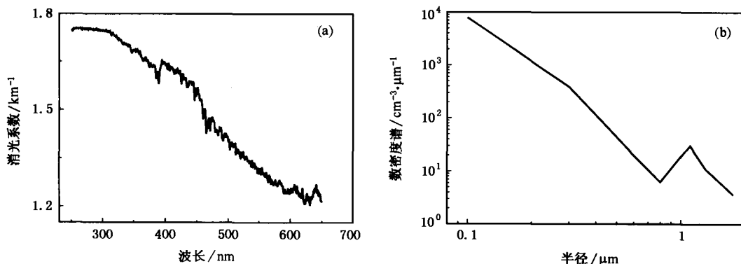
图 3 (a)2005 年 10 月 9 日 0:00 时测得的消光系数及(b)此时对应的气溶胶数密度谱
