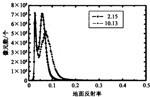
图 4 冬季(2002 年 2 月 15 日)和秋季(2002 年 10 月 13 日)的地表反射率—像元数二维曲线图
