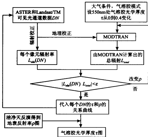
图 7 气溶胶光学厚度反演流程图 Fig. 7 Schematic diagram of AOT retrieval
