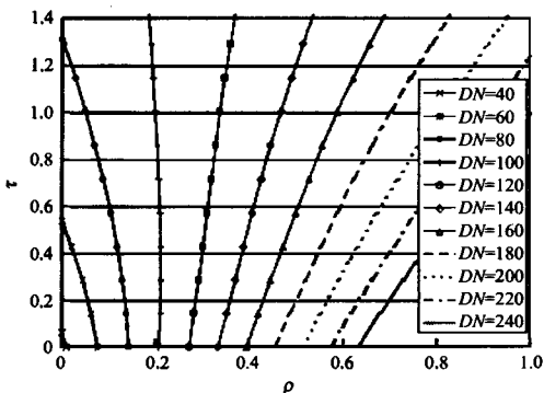
图 8 气溶胶光学厚度和地表反射率关系曲线图 (1999-01-14) Landsat/TM band1, 气溶胶模式乡村型 Fig. 8 Schematic diagram of AOT retrieval
