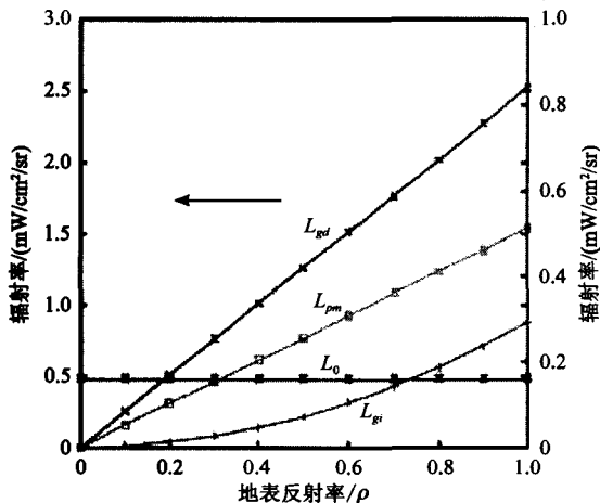
图 2 气溶胶光学厚度为 0.198 时,大气顶辐射,四个组成部分随地表反射率变化图( L_{gd} 的纵坐标在左边,其他三个组分的纵坐标在右边)
