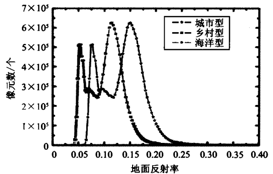
图 5 当气溶胶光学厚度为 0.34 时,在不同的气溶胶模式下,千叶地区春季 ASTER 波段 1 的地表反射率—像元数二维曲线图
