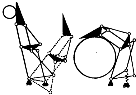
图4 包络抓取和精确抓取方式之间的切换
