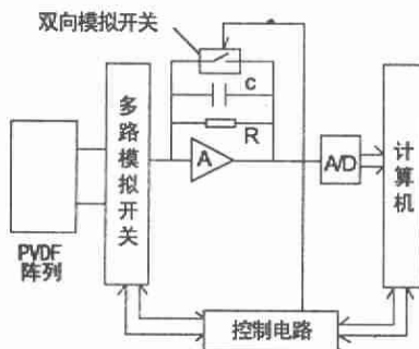
图10 接触力传感器信号采集电路
