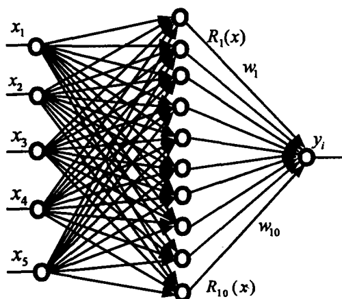
图8 基于RBF结构的模糊神经网络
