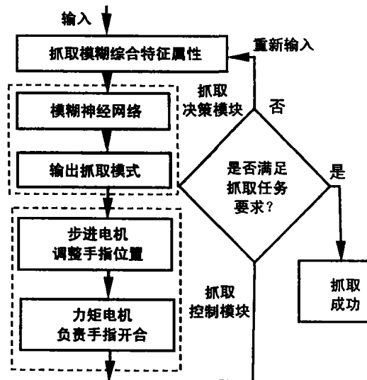
图7 欠驱动手爪自主抓取控制流程
