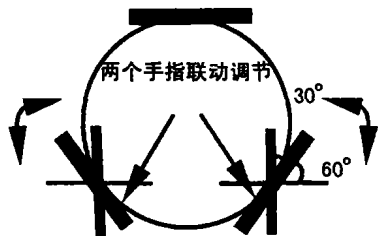
图5 欠驱动手爪调整手指位置形成多种抓取模式
