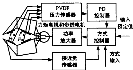
图9 基于传感器反馈的抓取控制结构
