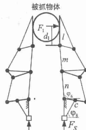
图 3 并行精确抓取机构 Fig. 3 The parallel precision grasp mechanism
