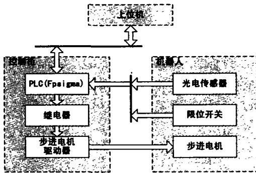
图7 控制结构图
