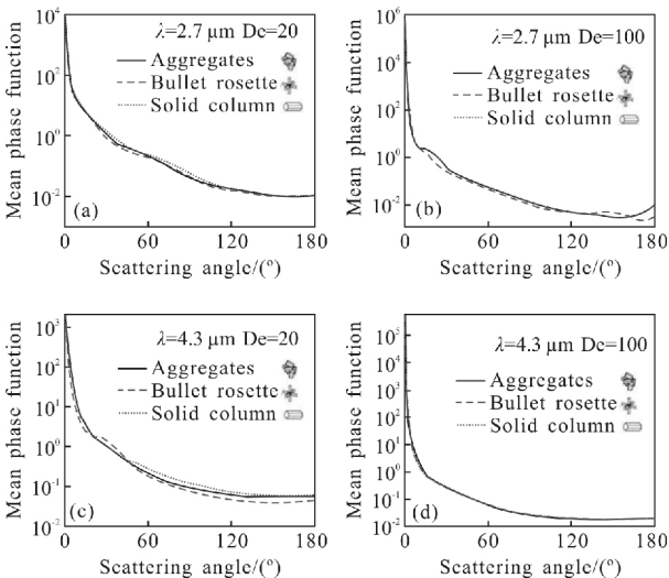
图 2 卷云 2.7 \mu\text{m} 和 4.3 \mu\text{m} 带平均散射相函数
