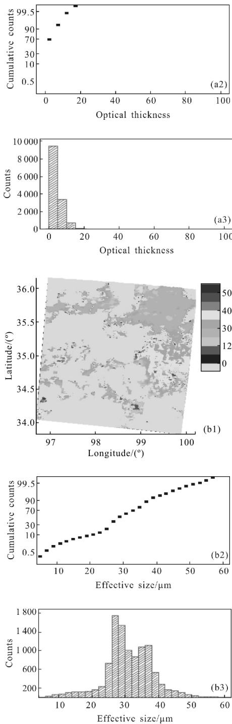
图 4 MODIS 实测的卷云光学厚度和有效尺度
