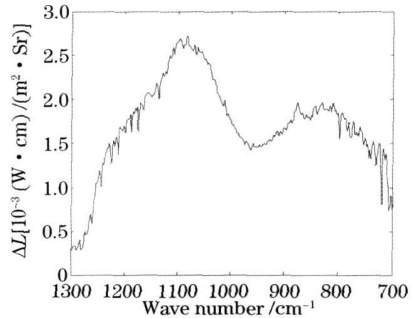
图 6 试验测量的高岭土粉末气溶胶红外光谱特征
