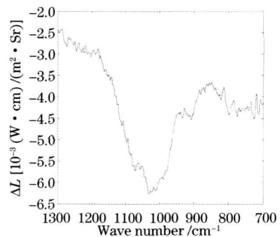
图 2 试验测量的生物孢子气溶胶红外光谱特征
