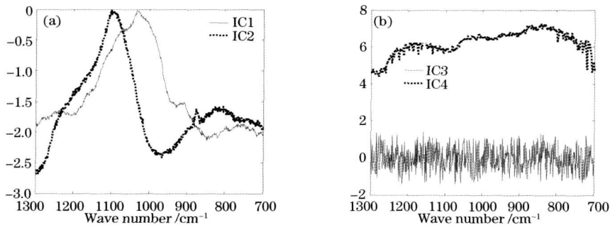
图 7 对图 6 所示的 ICA 分析得到的独立分量。(a) 红钱光谱特征, (b) 噪声和基线漂移
