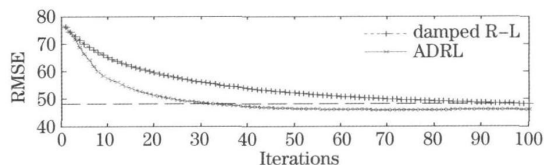
图 4 实验 2 的均方根误差
