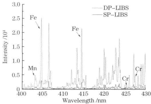
图 2 SP 和预烧蚀 DP 激发钢样的光谱图
