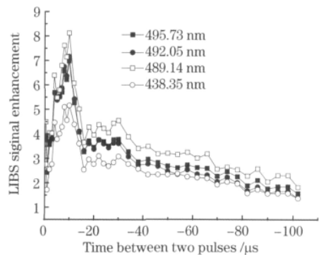
图 4 DP 激发的 4 条谱线的增强程度随 \Delta t 的变化 Fig. 4 LIBS emission enhancement versus \Delta t using pre-ablation double excitation for four lines
