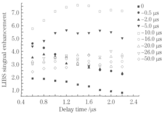
图 6 在不同的脉冲间隔下,信号的增强程度随采集延时变化
