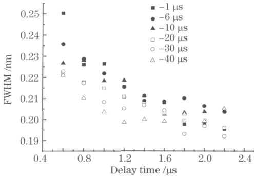
图 8 在不同的两脉冲间隔下,FWHM 随采集延时变化
