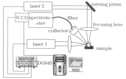
图 1 预烧蚀 DP-LIBS 实验系统示意图
