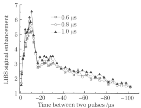
图 3 预烧蚀 DP 产生的发射谱线增强程度随 \Delta t 的变化
