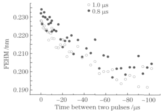
图 7 FWHM 随两激光脉冲间隔变化
