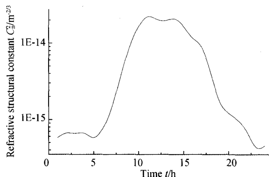
图 8 合肥七月份近地面湍流强度日变化趋势
