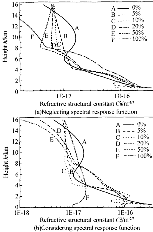
图4 反演结果 Fig. 4 Inversion results
