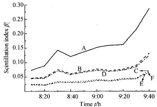
图6 闪烁指数随时间的变化趋势 Fig. 6 Curves of scintillation index vs time
