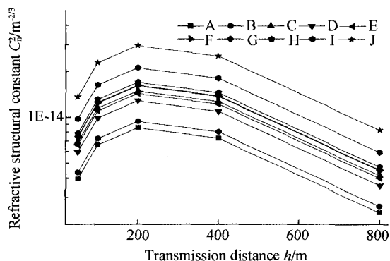
图 9 C_n^2 在传输路径上的分布曲线
