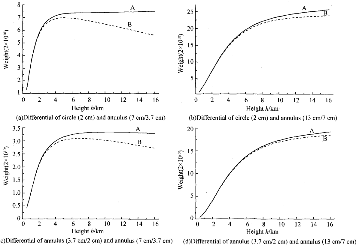
图 3 光谱响应函数对差分权重函数的影响
