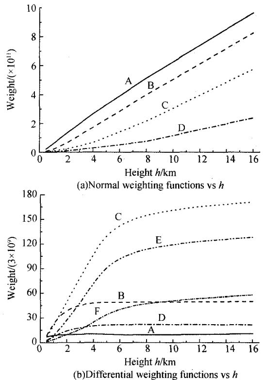
图 2 常规及差分权重函数随高度的变化曲线
