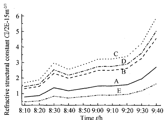
图 7 C_n^2 随时间的变化趋势
