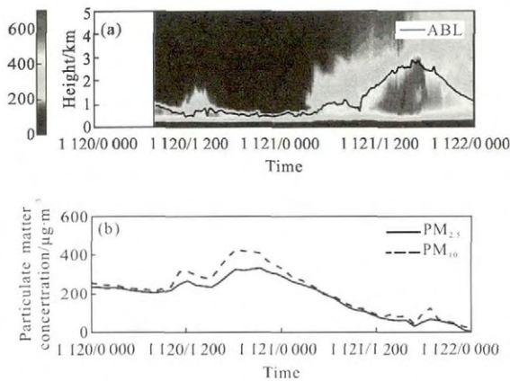
图 3 2014 年 11 月 20 日~2014 年 11 月 21 日 TWAR 连续测量的大气边界层时空分布(a)以及 PM 质量浓度(b)的变化 Fig.3 Continuous observation of ABL (a) by TWAR and variation of PM concentrations (b) form 20 Nov 2014 to 21 Nov 2014
