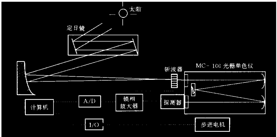
图 1 太阳光谱测量系统示意图
