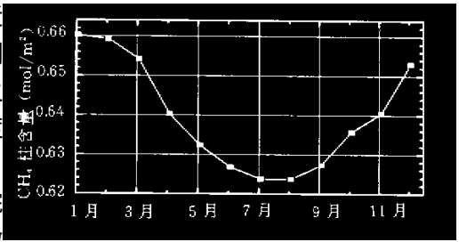
图 7 合肥地区 1997~1998 年 甲烷柱含量的月平均变化
