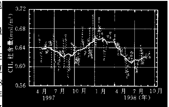
图6 1997年4月至1998年9月18日合肥地区甲烷柱含量的日平均值随时间的变化(实线为30d的滑动平均)
