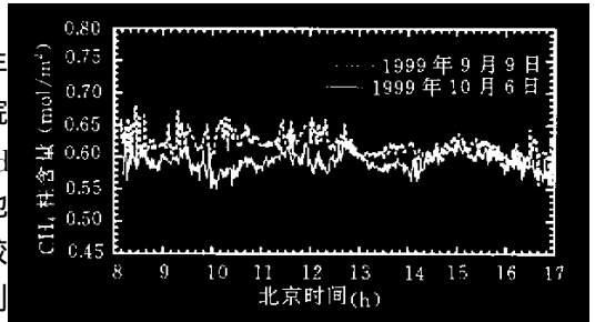
图5 1997年9月9日和10月6日甲烷柱含量随时间的变化
