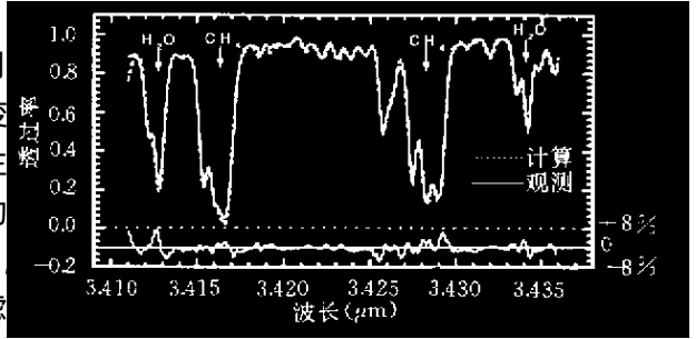
图4 1998年5月16日14时01分测量的太阳光谱(实线)与计算结果(虚线)的比较
